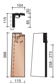
7020 LINKER HALVE GEVELPAN
