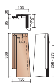
7030 RECHTER HALVE GEVELPAN
