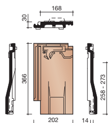
8640 VENTILATIE- /HAAKDOORVOERPAN MET ROOSTER 10CM 2
