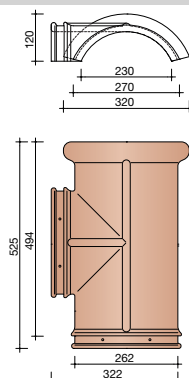
VERBINDINGSSTUK TUSSEN 3 VORSTEN
