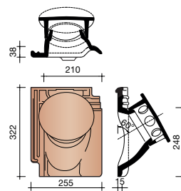
8741 DOORVOERPAN 100 MM MET AANSLUITMODULE
