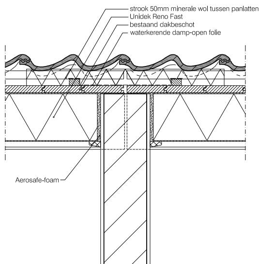
Detailtekening 1 - Woningsscheidende wand Unidek Reno Fast
