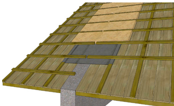
Figuur 10 - Detail woningscheidende wand
