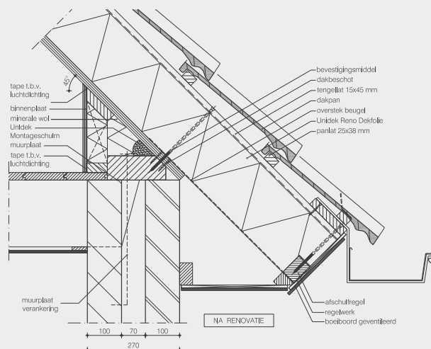
Detailtekening 3 - Overstek met horizontale aftimmering
