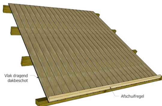
Figuur 1 - Detail afschuifregel op vlak dakbeschot
