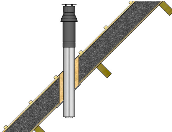
Figuur 14 - Detail sparring mantelbuis
