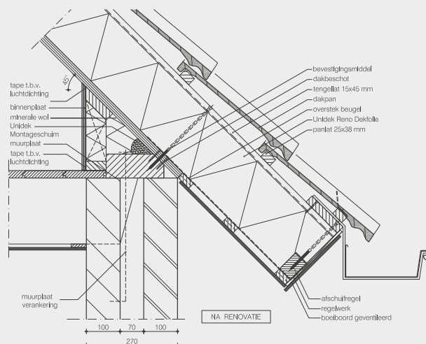
Detailtekening 2 - Overstek met aftimmering evenwijdig aan het dakelement
