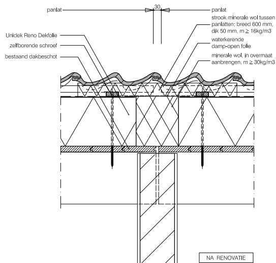
Detailtekening 1 - Woningscheidende wand Unidek Reno Dekfolie
