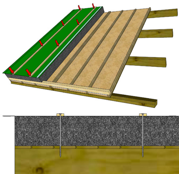
Figuur 9 - Bevestigingspunten
