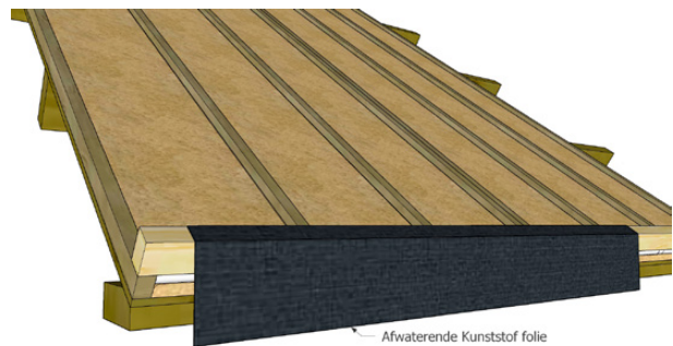
Figuur 6 - Afwaterende kunststof folie
