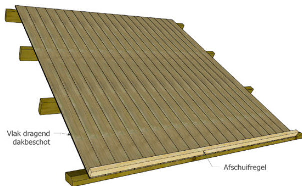
Figuur 4 - Afschuifregel op vlak dragend dakbeschoot
