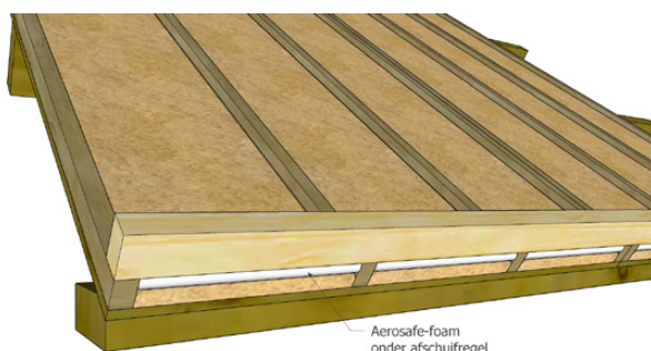
Figuur 5 - Aerosafe-foam onder afschuifregel
