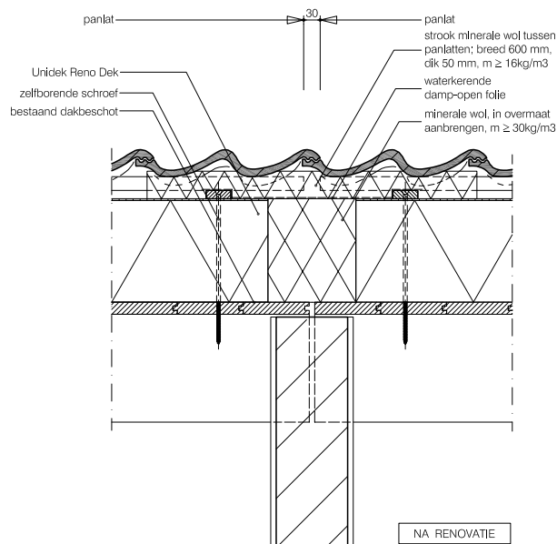
Detailtekening 1 - Woningsscheidende wand Unidek Reno Dek
