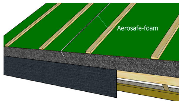
Figuur 9 - Unidek Aerosafe-foam verticale naden
