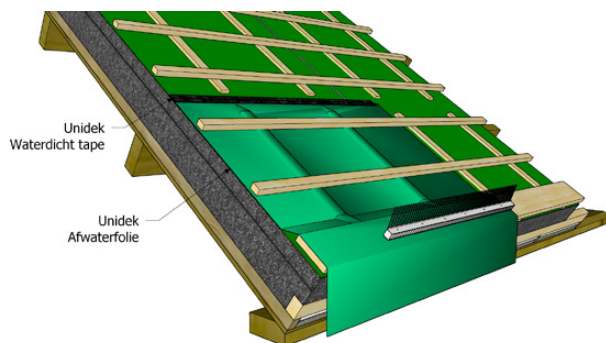
Figuur 11 - Detail gootafwatering met Unidek Afwaterfolie en Unidek Waterdicht tape
