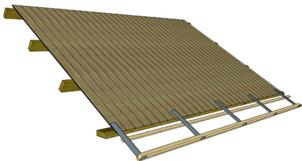
Figuur 10 - Unidek Overstekbeugel
