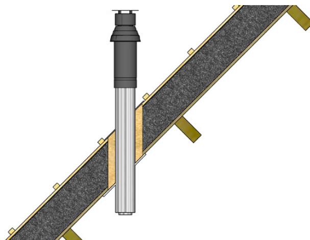
Figuur 13 - Detail sparring mantelbuis
