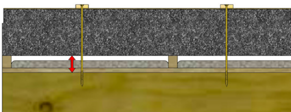
Figuur 8 - Detail extra schroeflengte
