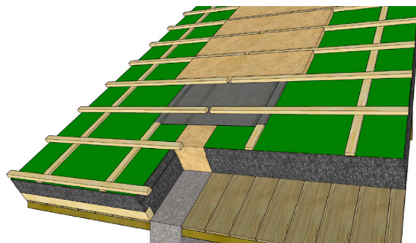
Figuur 12 - Detail woningscheidende wand
