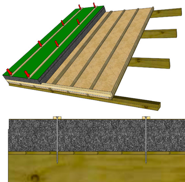
Figuur 7 - Bevestigingspunten
