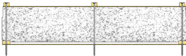
Figuur 5 - Detail bevestiging Unidek Aero Light RE
