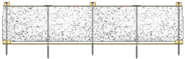
Figuur 6 - Detail extra bevestiging
