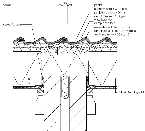
Detailtekening 1 - Woningsscheidende wand Unidek Aero Light RE
