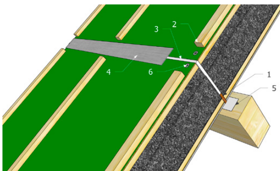
Figuur 9 - Detail horizontale naden
