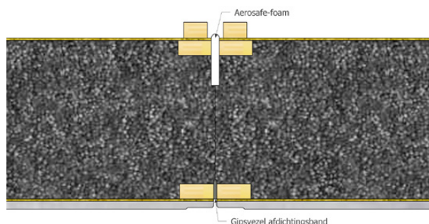
Figuur 7 - Detail Aerosafe-foam en Gipsvezel afdichtingsband
