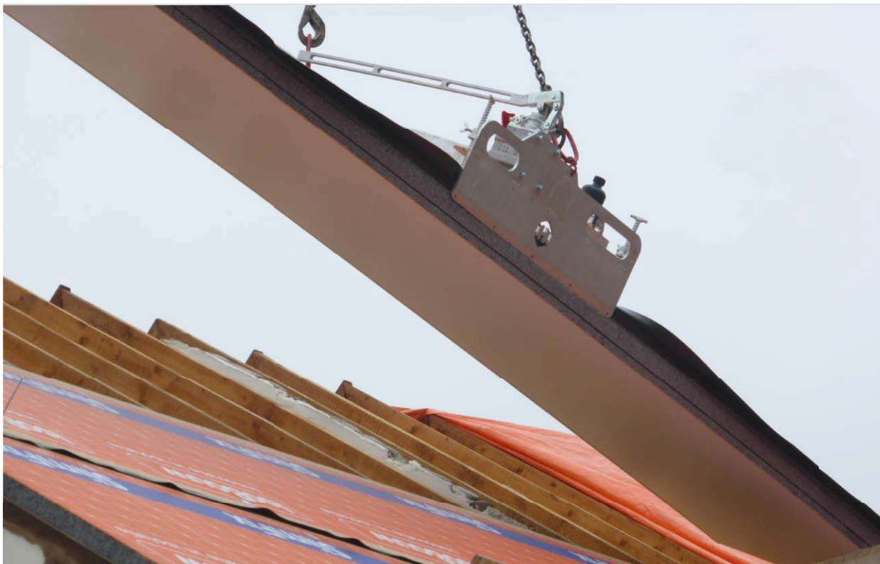
Te monteren met een HTZ dakplatenklem
