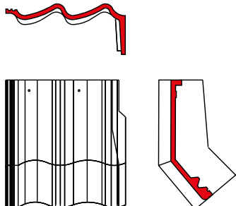
knikgevelpan rechts 140°
