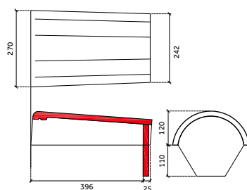
uni-eindvorst
