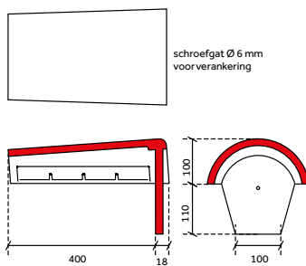
uni-beginvorst
