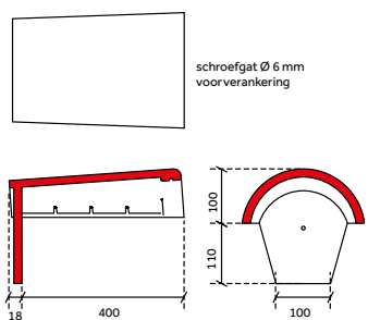
uni-eindvorst
