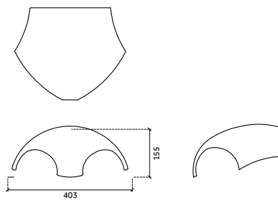
3-zijdig broekstuk
