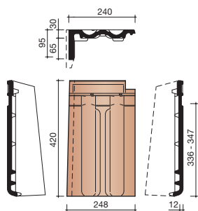
7080 LINKER GEVELPAN
