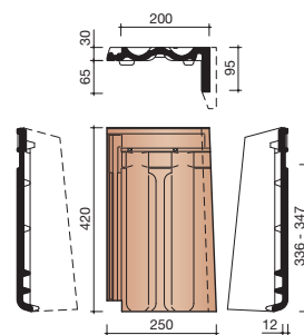
7090 RECHTER GEVELPAN
