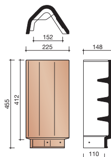
2200 CHAPERONVORST
