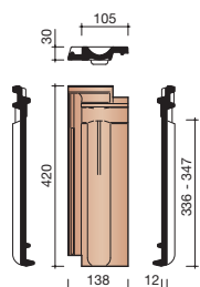
8010 HALVE PAN
