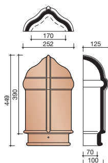
1360 EZELSRUG BEGINKEPERVORST
