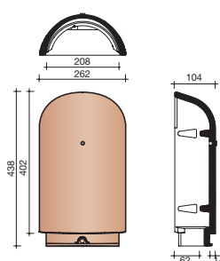
1061 HALFRONDE BEGINKEPERVORST
