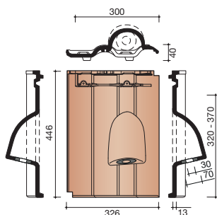
8958 KABELDOORVOERPAN MET NEOPREEN-RING
