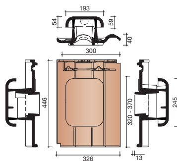
8741 DAKDOORVOER INCL. AANSL. Ø 100 MM
