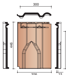
8640 VENTILATIE- / HAAKDOORVOERPAN MET ROOSTER 29CM 2
