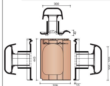
8728 DAKDOORVOER INCL. AANSL. Ø 125 MM
