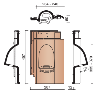
8660 GIERZWALUWPAN
