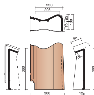
7590 RECHTER GEVELCHAPERONPAN
