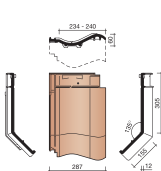
8200 KNIKPAN
