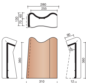
7580 LINKER GEVELCHAPERONPAN
