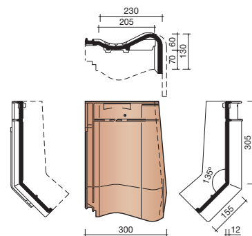
7290 RECHTER GEVELKNIKPAN
