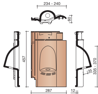
8655 MUSSENPAN
