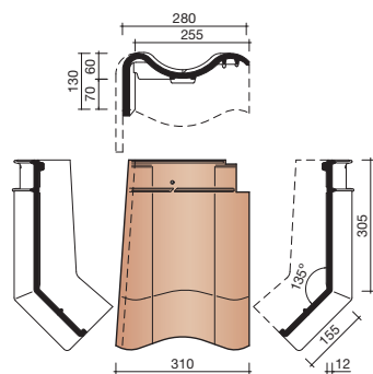
7280 LINKER GEVELKNIKPAN
