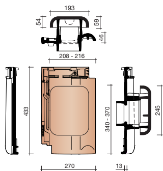
8741 DAKDOORVOER INCL. AANSL. Ø100 MM
