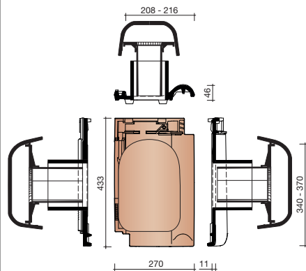
8728 DAKDOORVOER INCL. AANSL. Ø125 MM
