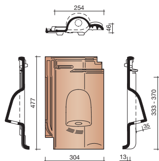
8655 MUSSENPAN
