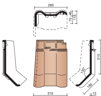
7280 LINKER GEVELKNIKPAN
