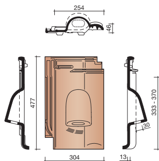
8660 GIERZWALUWPAN
