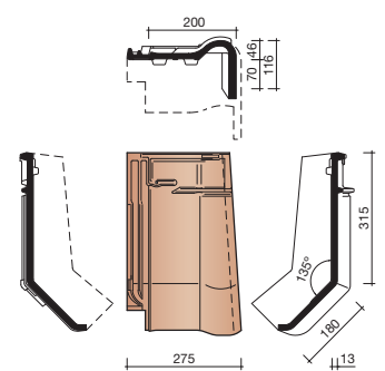
7290 RECHTER GEVELKNIKPAN
