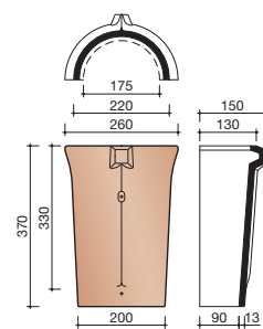
3100 SCHUBVORST
