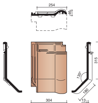
8200 KNIKPAN
