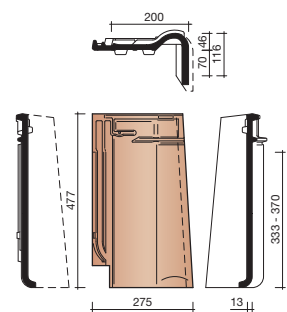
7090 RECHTER GEVELPAN
