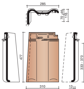
7080 LINKER GEVELPAN
