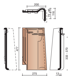
8540 GEVELAANSLUITPAN RECHTS
