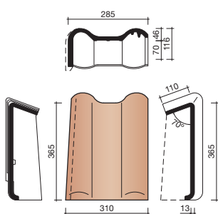
7580 LINKER GEVELCHAPERONPAN
