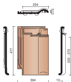
0000 ALEGRA 10 DAKPAN
