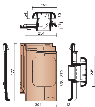
8741 DAKDOORVOER INCL. AANSL. Ø100 MM
