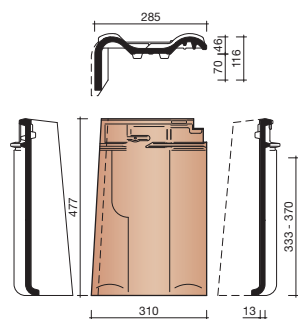
8545 GEVELAANSLUITPAN LINKS
