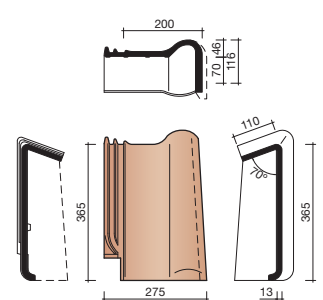
7590 RECHTER GEVELCHAPERONPAN
