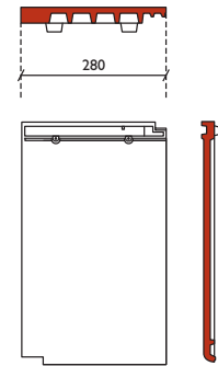
linker eindpan
