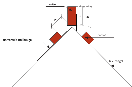
nokbeugel geknikt op perforatie
