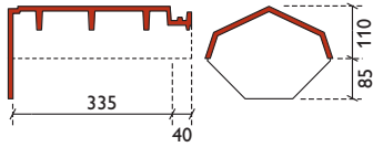
HV topgevelbeginvorst type K
