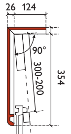
chaperonpan 90° (gezaagd)
