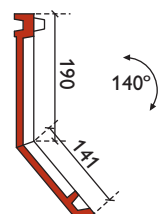
knikpan 140° (gezaagd model)
