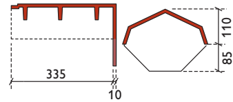
HV topgeveleindvorst type K
