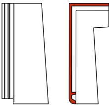
halve chaperongevelpan 90° rechts
