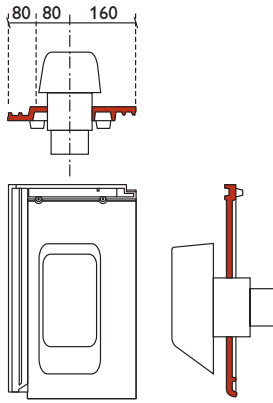
ontluchtingspan
