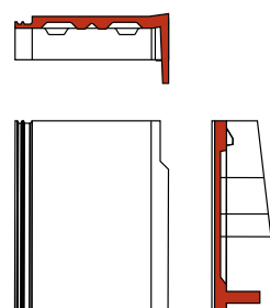
gevelonderpan rechts
