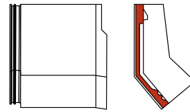
knikgevelpan 140° rechts
