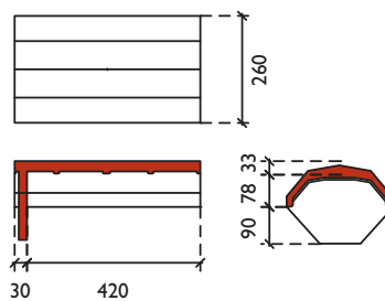
HV sluitvorst
