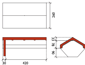
hoekige sluitvorst
