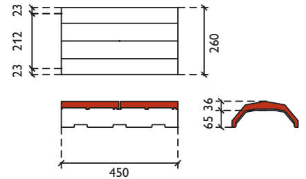
HV vorst
