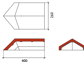
hoekige hoekkeperbeginvorst
