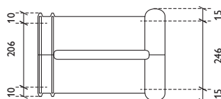
doorvoerpan (met doorvoer voor dakhelling 25° – 45°)
