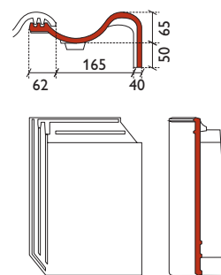
gevelpan rechts
