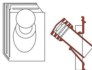
doorvoerpan (met doorvoer voor dakhelling 25° – 45°)
