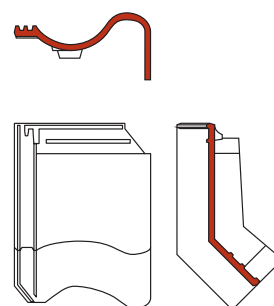
knikgevelpan rechts
