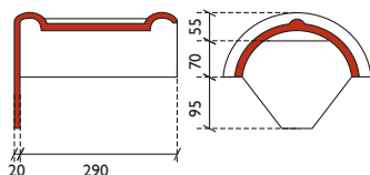
halfronde topgeveleindvorst model Tegelen
