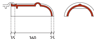
halfronde hoekkeperbeginvorst model Tegelen
